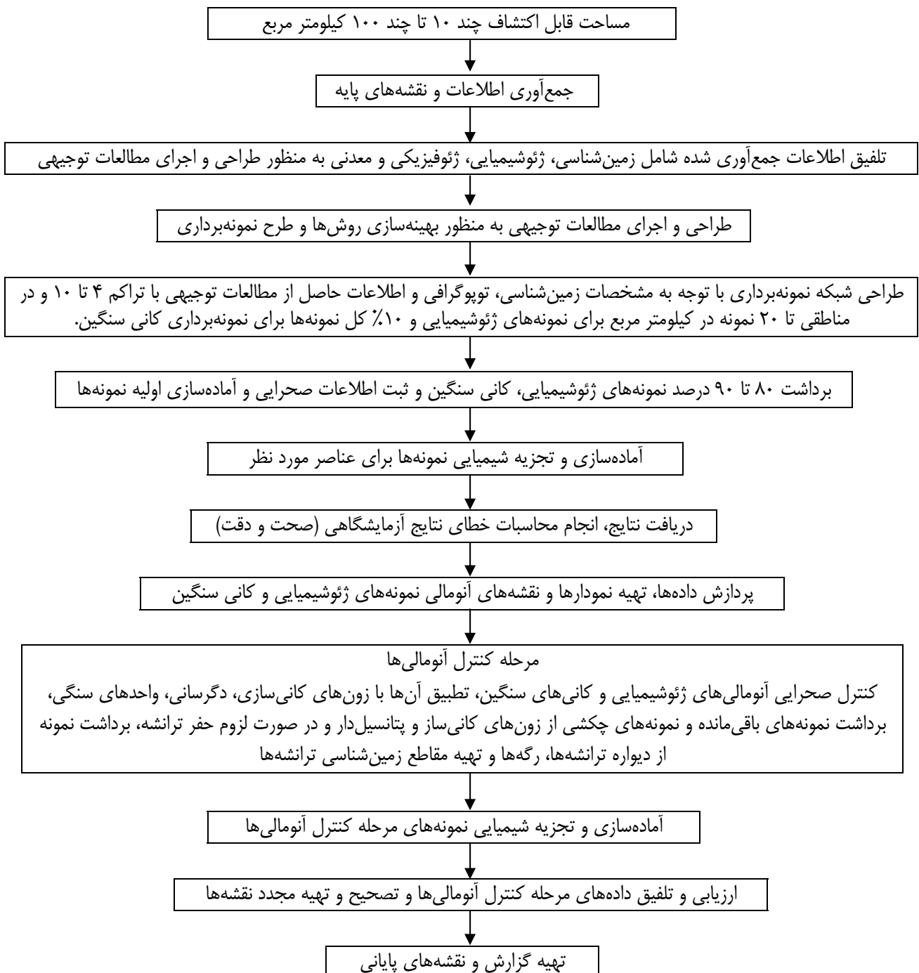
شکل ۱-۲ - نمودار جریانی اکتشاف ژئوشیمیایی آبراهه‌ای.
